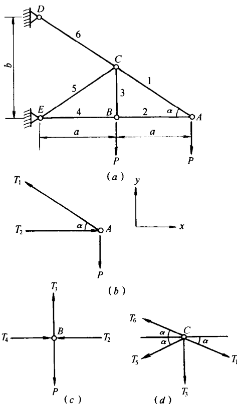
图 5-6 节点法解简单桁架
