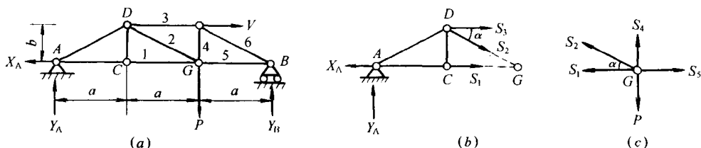
图 5-7 截面法解桁架受力
