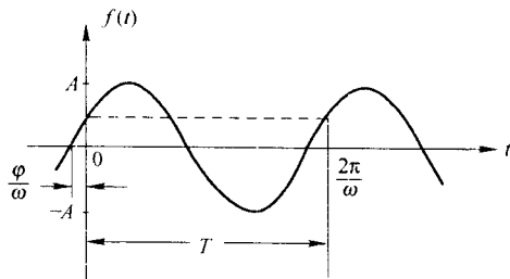
图 1-9 正弦信号
