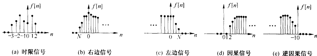
图 1-7 离散时间信号的几种情况
