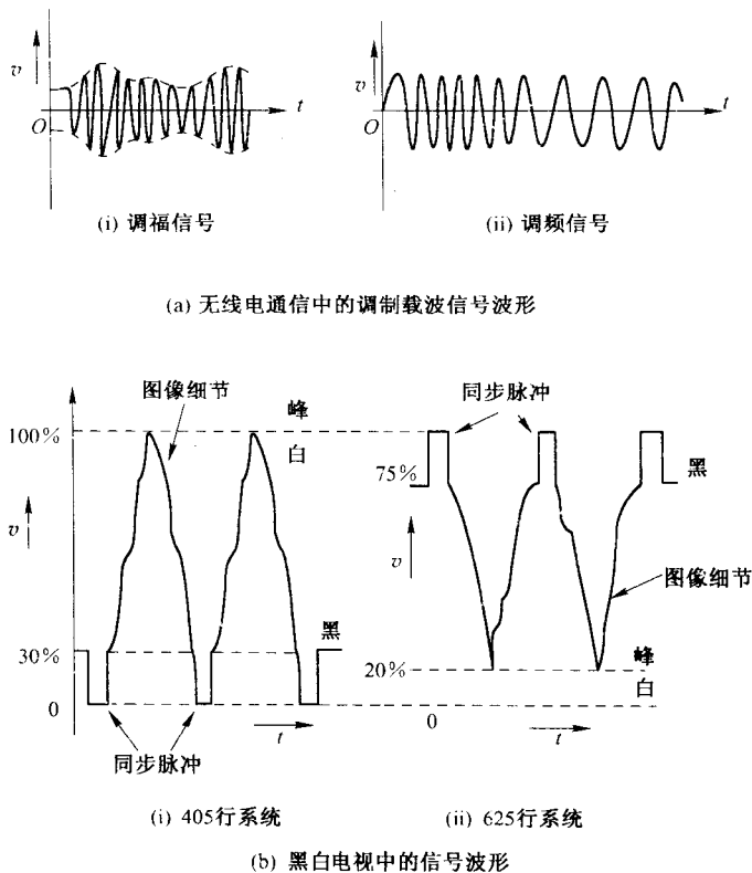
图 1-8 用于无线电通信和电视的几种信号波形
