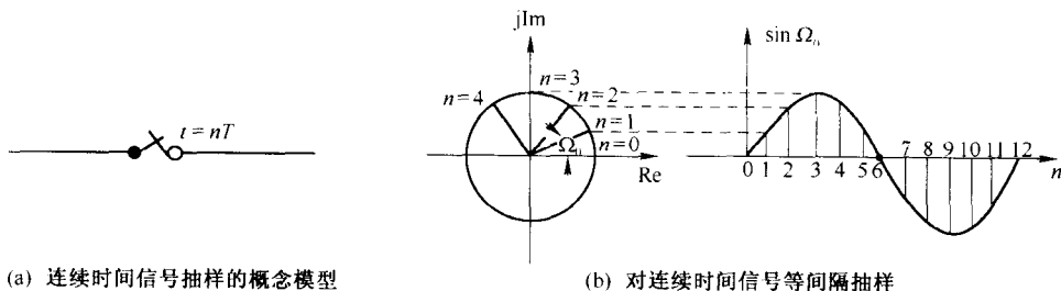
图 1-5 对连续时间信号等间隔抽样概念示意图
