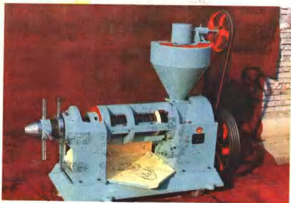
图12 雅安青江机器厂生产的部优名产——蒙山牌 6 YL-95型螺旋榨油机
