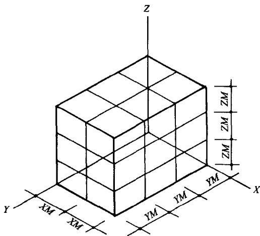
图 1-3 模数化空间网格
