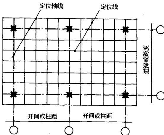
图 1-4 定位轴线和定位线
