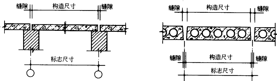
图 1-5 标志尺寸与构造尺寸的关系
