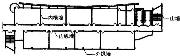
图 2-1 不同位置方向的墙体名称
