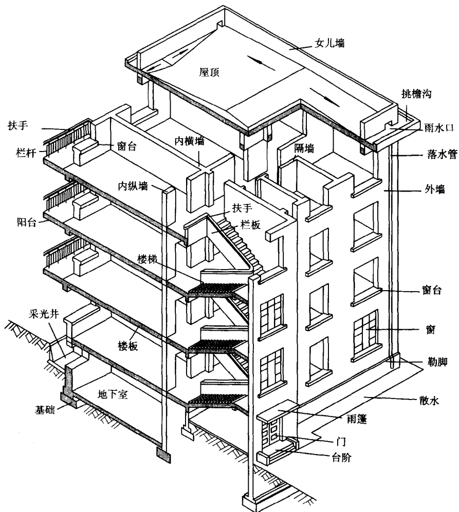
图 1-1 墙体承重结构的建筑构造组成
