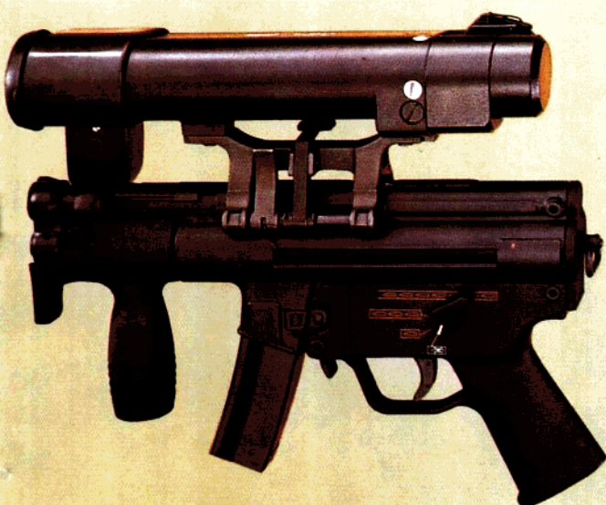
图127(a) 德国 9 mm MP5 KA4 式冲锋枪
