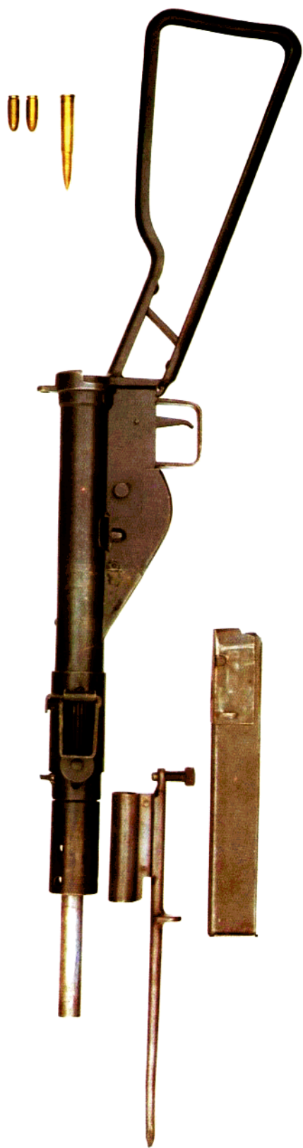
图81 英国 9mm 司登 MK II 式冲锋枪
