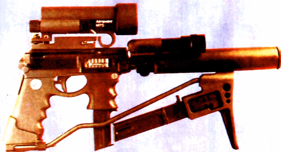
图95 英国9mm 布希曼冲锋枪
