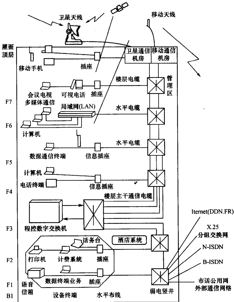
图 1-2 综合布线系统与信息通信网络的连接关系
