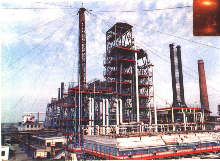
◁ 抚顺石油三厂的设备档案在生产中发挥了巨大作用，图为该厂40万吨 / 年加氢裂化装置
