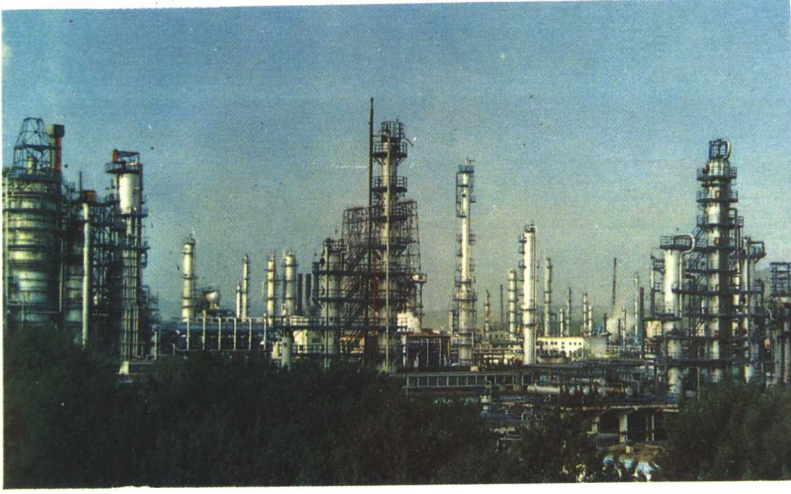
◁科技档案完整准确的抚顺石油二厂
