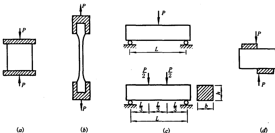
图 1.3 材料所受外力示意图
