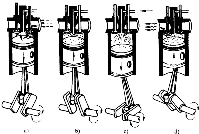
图 2-8 单缸四行程柴油机的工作过程
