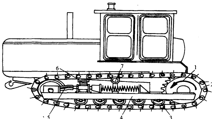
图 2-3 履带式拖拉机行走系统的组成
