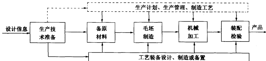
图 1-1 产品的制造过程
