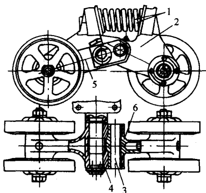
图 2-4 支重台车架
