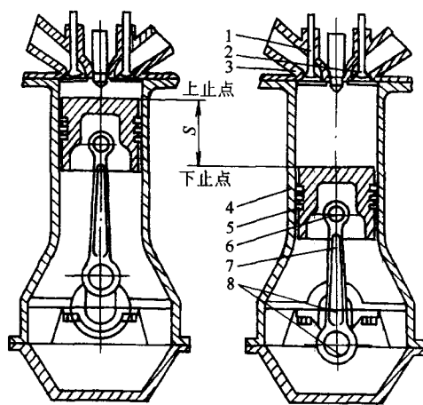
图 2-7 单缸四行程柴油机的机械简图
