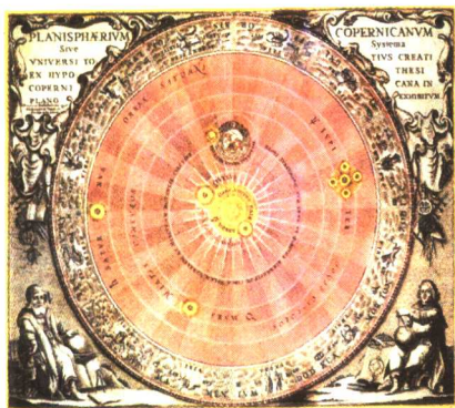
《天体运行论》一书中的“日心说”示意图。水星、金星、地球、火星、木星、土星由近及远地围绕太阳旋转，月球围绕地球旋转
