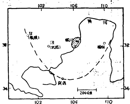
图1 1477年银川地震等震线图
