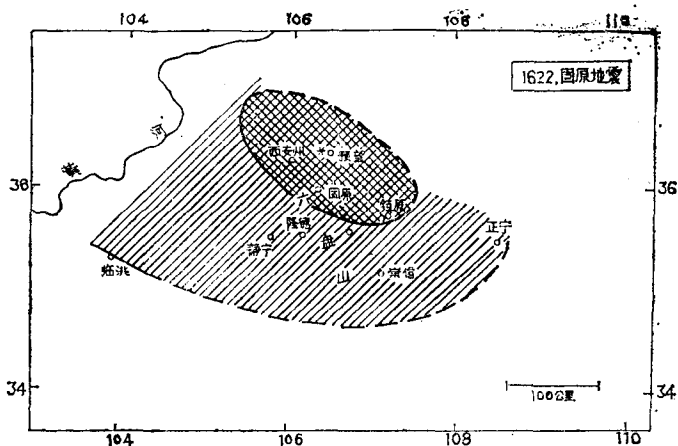
图 3 1622年固原地震等震线图
