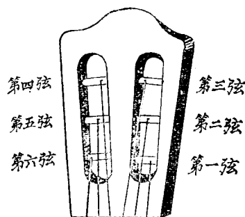
夏威夷吉他系弦图
