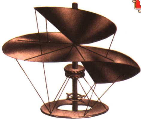
达·芬奇设计的直升机的螺旋桨模型
