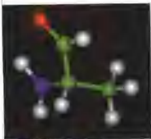
一种氨基酸分子结构模型。
