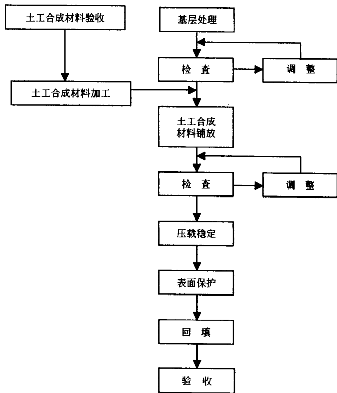
图 1.1.6.1 土工合成材料地基施工工艺流程
