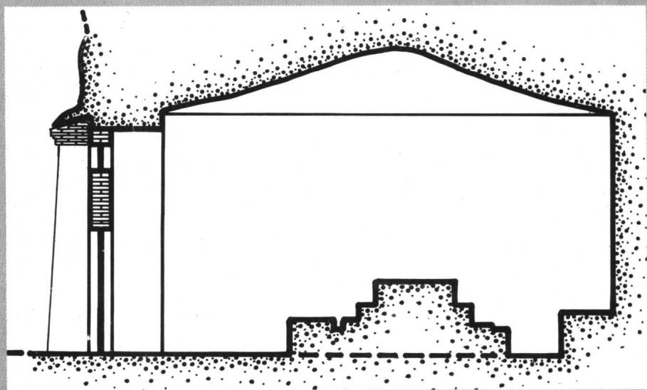
剖面示意图
