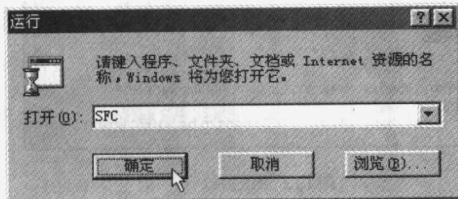
图1.5 “运行”对话框
