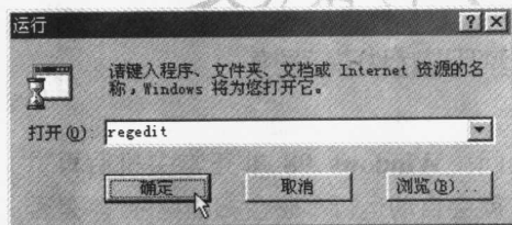
图1.8 “运行”对话框
