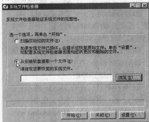
图1.6 提取文件
