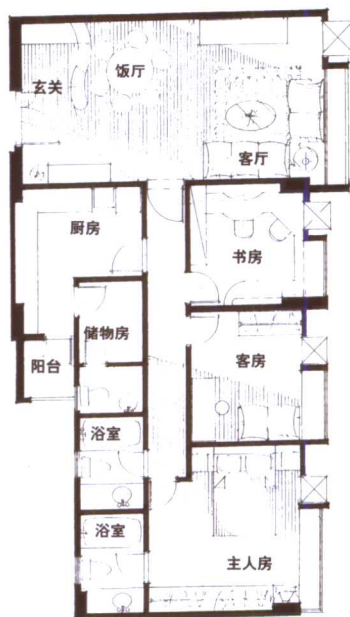
平面设计图
