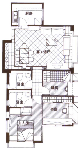
平面设计图
