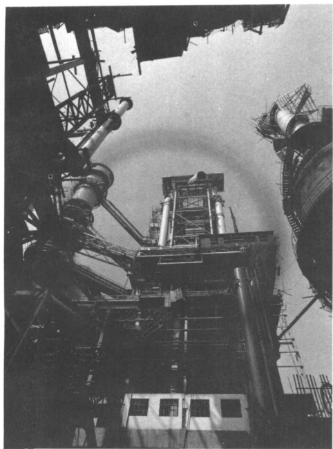
马钢兴建的2500立方米大高炉雄姿。
