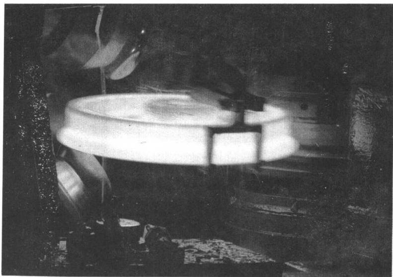
马钢正在轧制中的火车轮箍。
