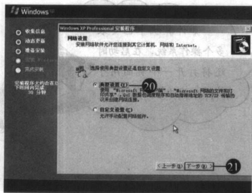
图 1-15 设置网络
