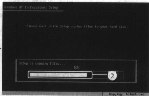
图 1-2 复制文件
