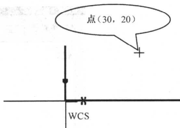
图 1-4 绘制点 (30, 20)
