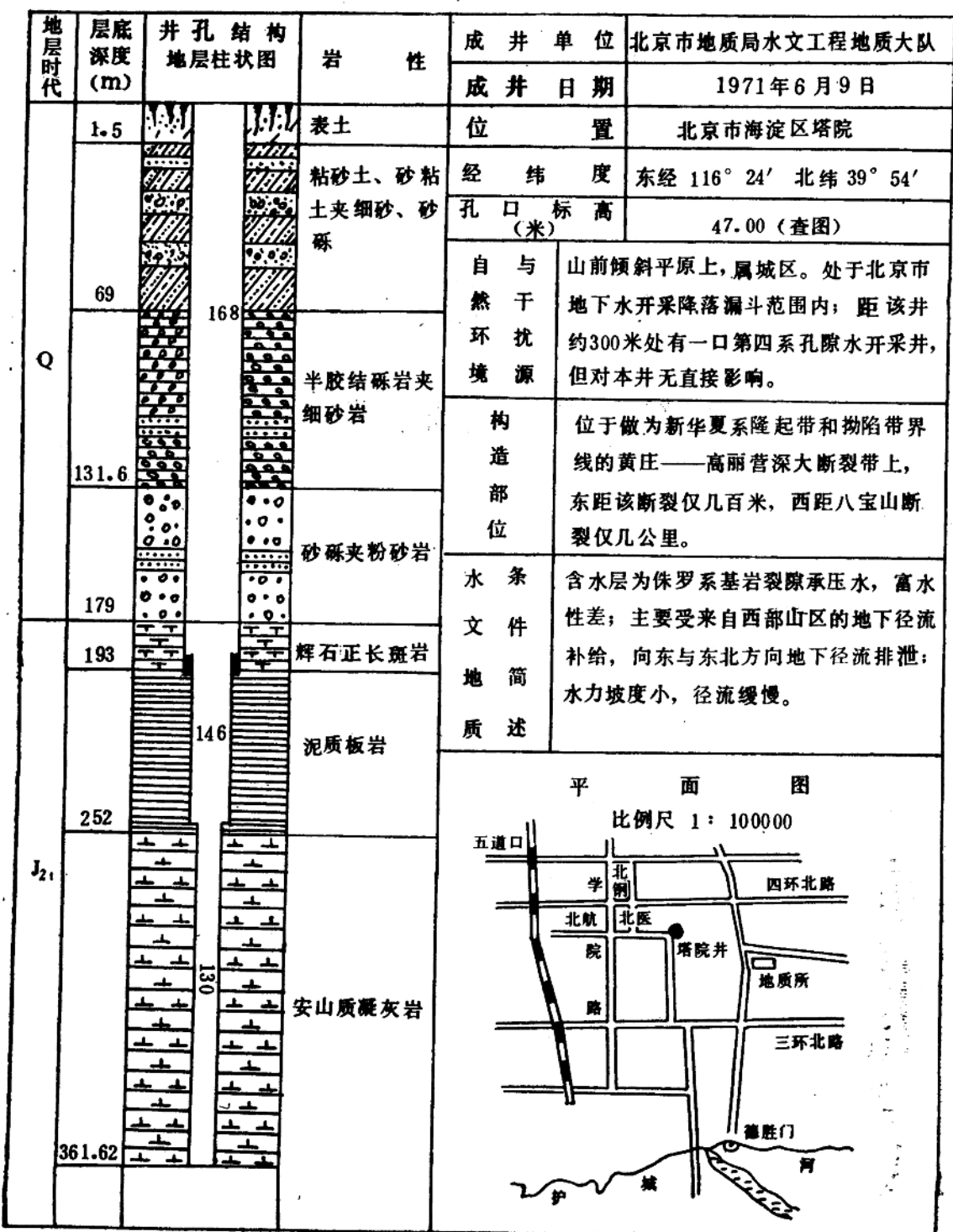
塔院井孔地质柱状图
