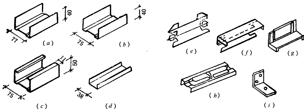
图 1-1-1 C75 系列龙骨主件和配件示意
