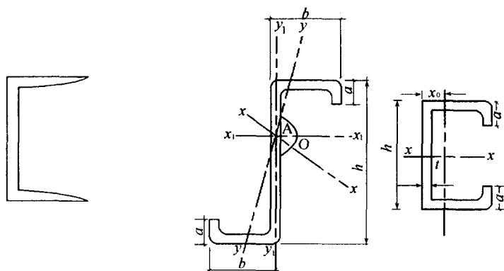
图 1-1-4 槽钢截面示意
