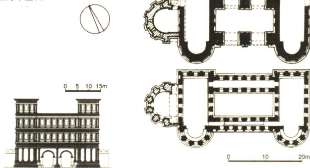
黑门平面图
