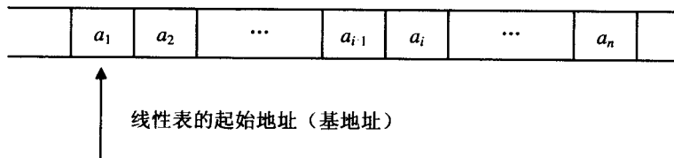
图 1.2 线性表的顺序存储结构示意图
