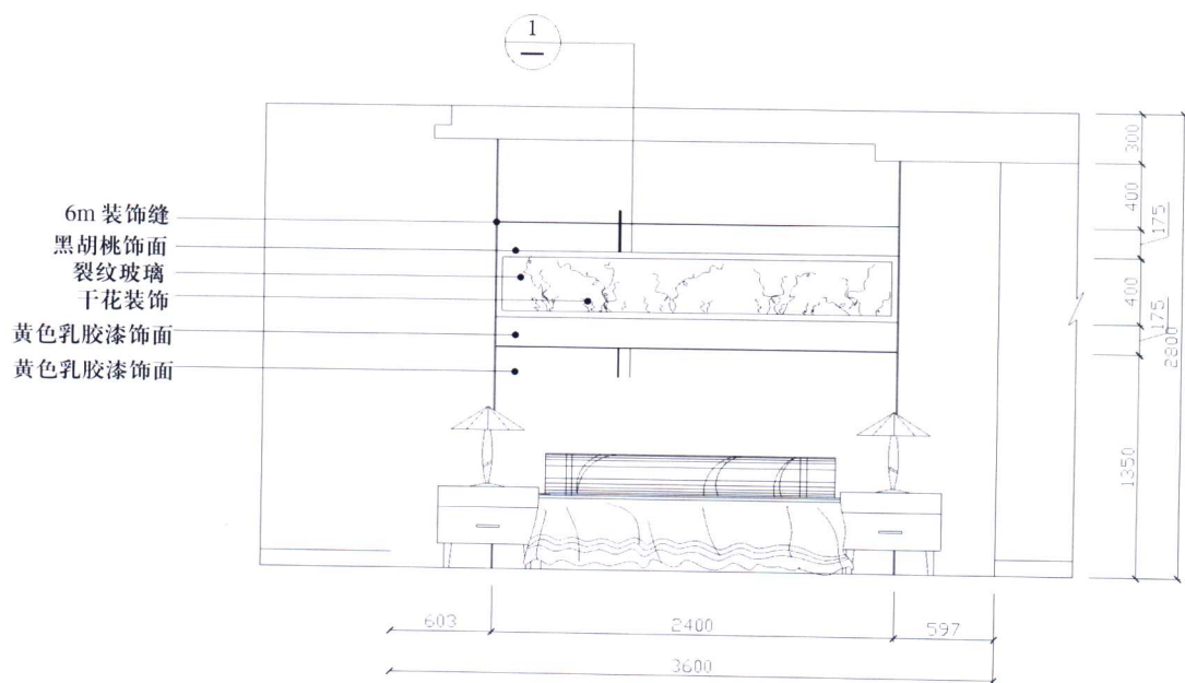
卧室床背景立面图
