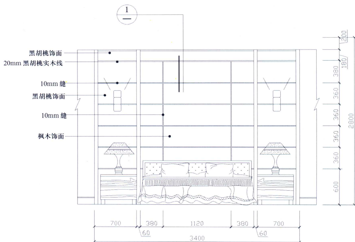
卧室床背景立面图
