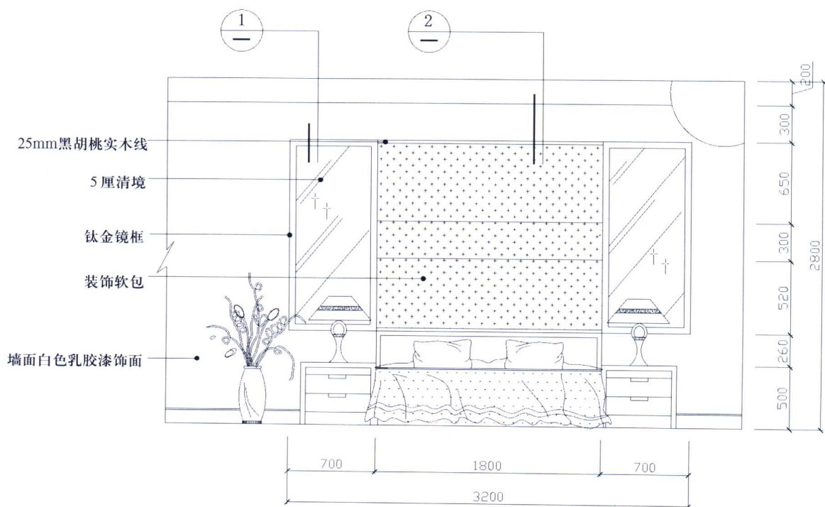
卧室床背景立面图
