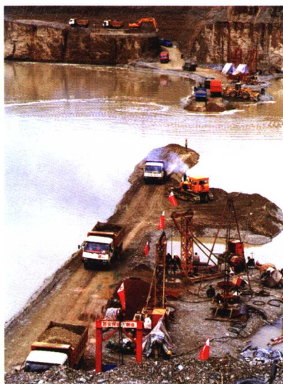
通天河大桥桥墩基础施工
