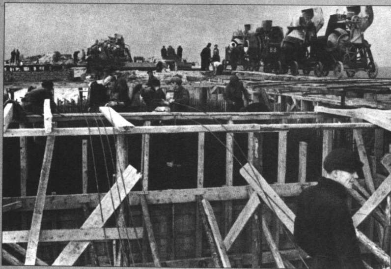
法国劳工正准备将混凝土浇灌到木头模子中,以建造钢筋加固的碉堡城墙。
