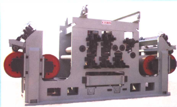
两弯两矫带钢拉矫机: 整体式、分体式
