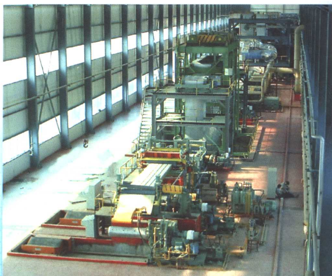
带钢热镀锌、彩涂生产线
