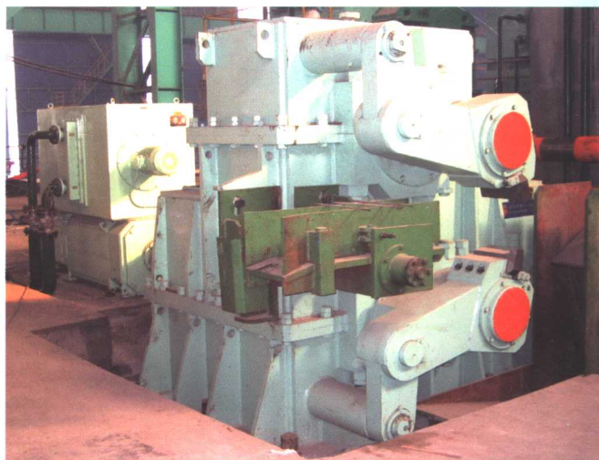
起停式飞剪机，剪切力 30t~160t；冷飞剪 450t
