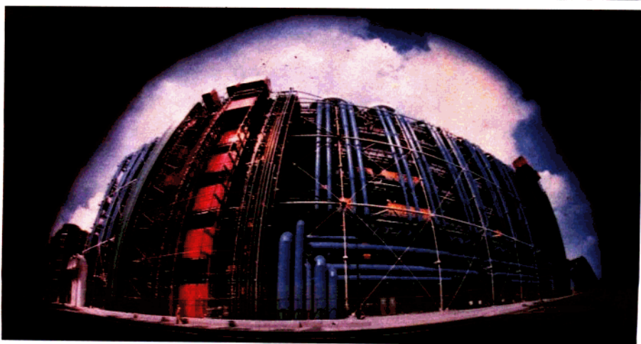
巴黎蓬皮杜文化中心(法国) 1977年 (意) 皮阿诺(英) 罗杰斯设计
