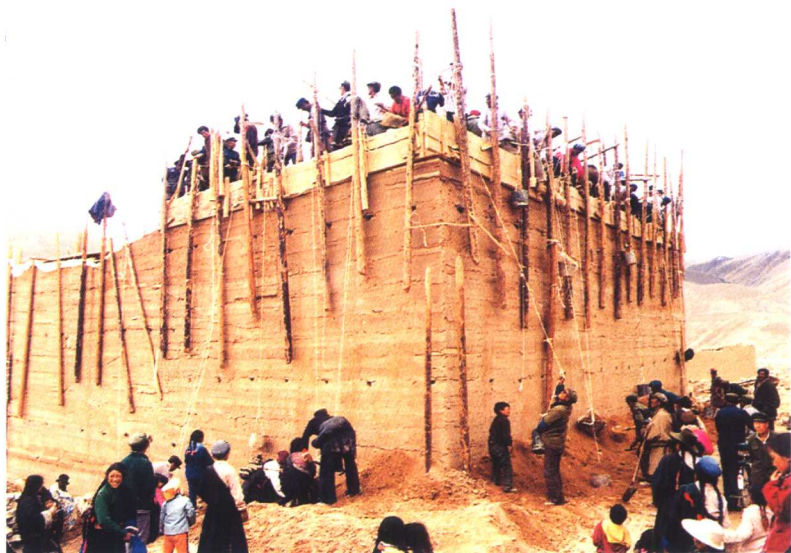
建筑工艺：板筑高墙施工场景
