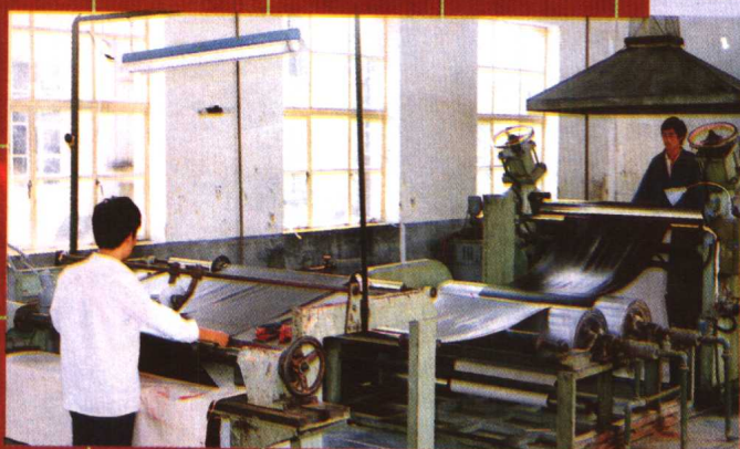
▲拉力试验机
