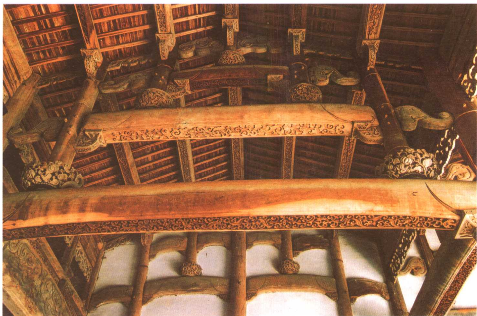
彩图 37 婺源汪口俞氏宗祠建于乾隆年间,为省文物保护单位。享堂望砖下,宏大的木构架叠罗汉似地直达屋顶:檩间饰一排云纹花板,梁、檩底面刻压地隐起花,平盘斗、丁头拱满施雕刻。
