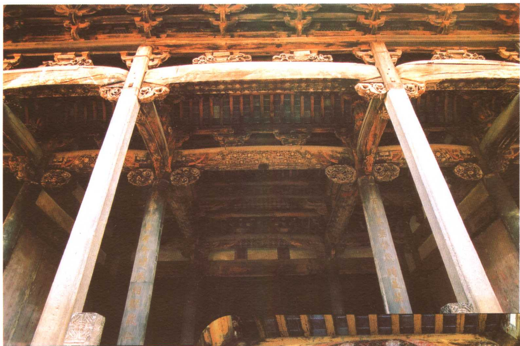
彩图 28 宝纶阁屋檐下斗拱挑头前各装有一对镂雕枫拱，柱子左右各装有一对雀替，肃穆的殿堂内像张开了对对将欲腾飞的翅膀，使静止的建筑显得轻盈而有生气。
