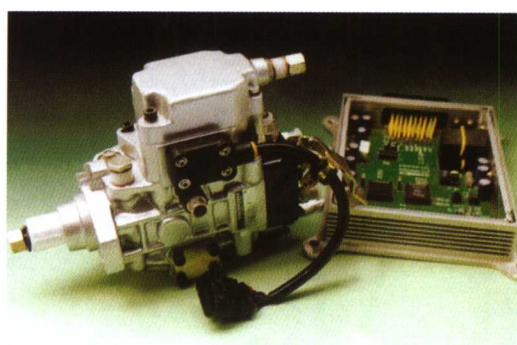
电控 VE 分配泵
