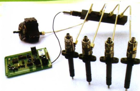
高压共轨
