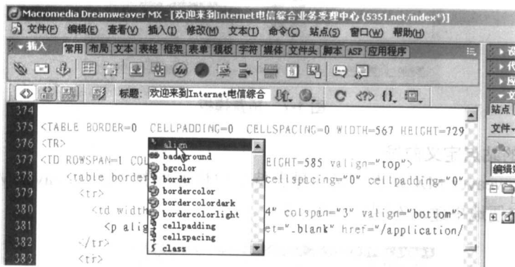
图 1-10 代码提示
