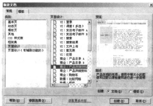
图 1-7 预置模板
