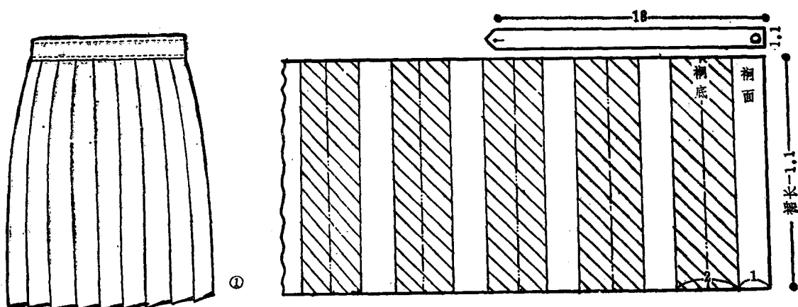
① 顺风裯裙
