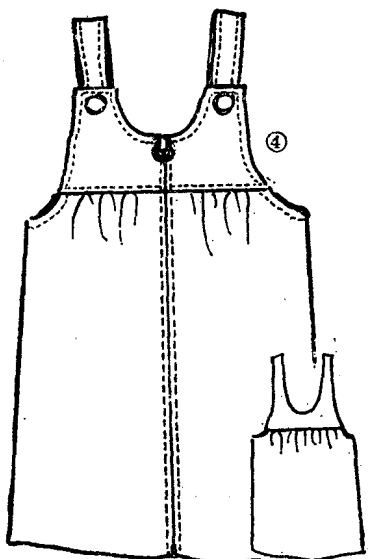
④这条两接式的吊带裙，前后裙片的接缝处收有绉裥，前面用拉链开襟，主要是为装饰。
