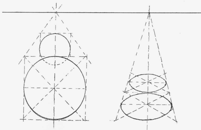
画椭圆的方法
