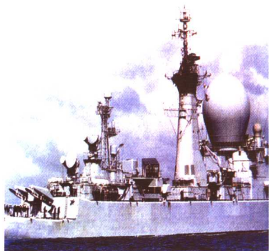
法国DRBI-23型雷达，用作对空对海的搜索
