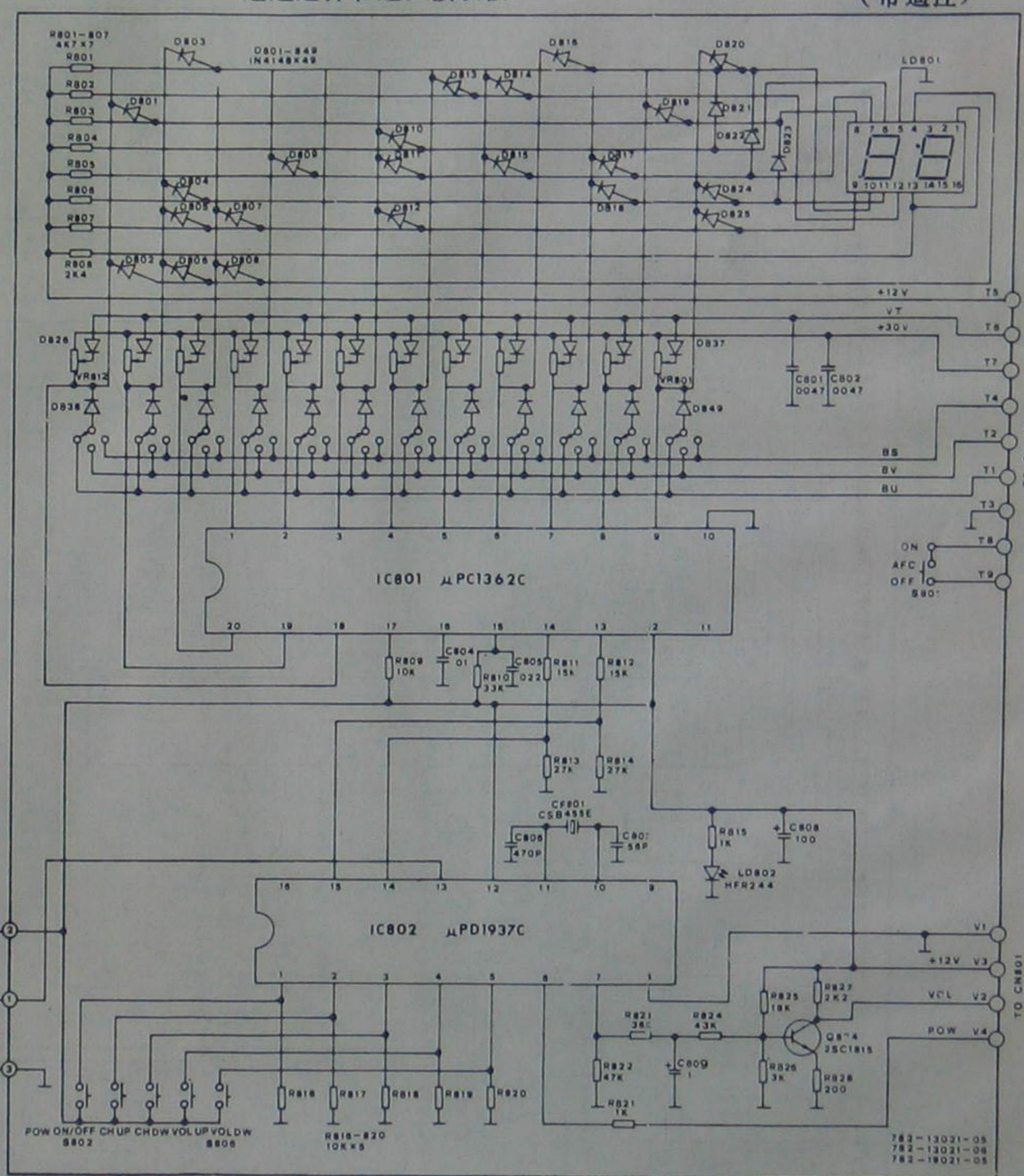
通道选择和遥控接收板
