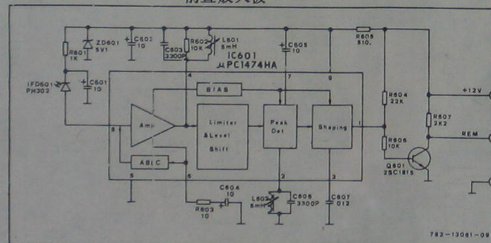
前置放大板
