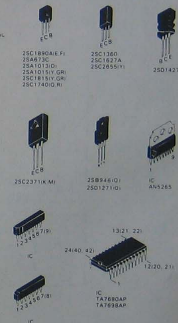
■晶体管和集成电路的引线图
