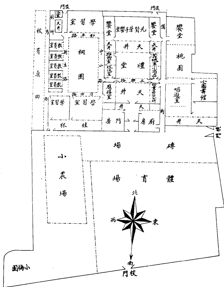
公益小學校舍平面圖之二 (一九三四年)
