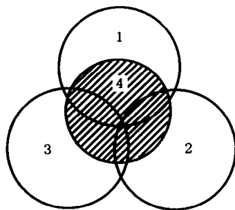
1. 大气圈 2. 水圈 3. 岩石圈 4. 生物圈
