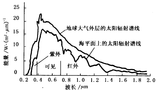
图 1-2 太阳发射光谱图
