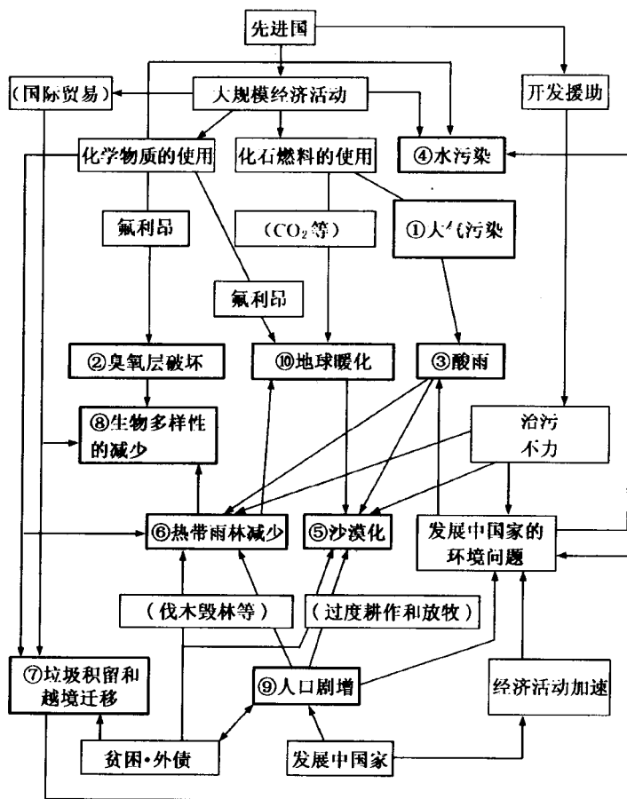
图 1-4 由人为原因引起的十大环境问题
