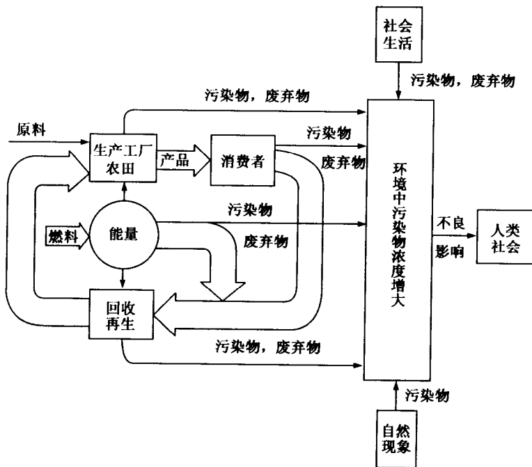
图 1-5 环境污染概念图
