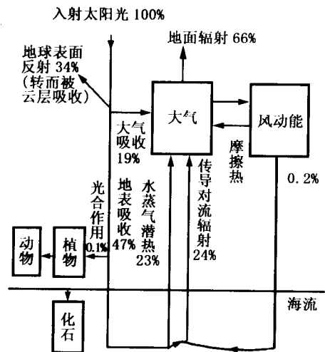
图 1-3 太阳能的流动
