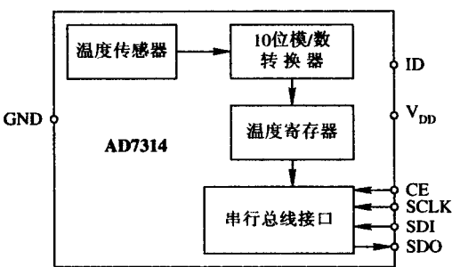
图 1.2 AD7314 的内部原理简图
