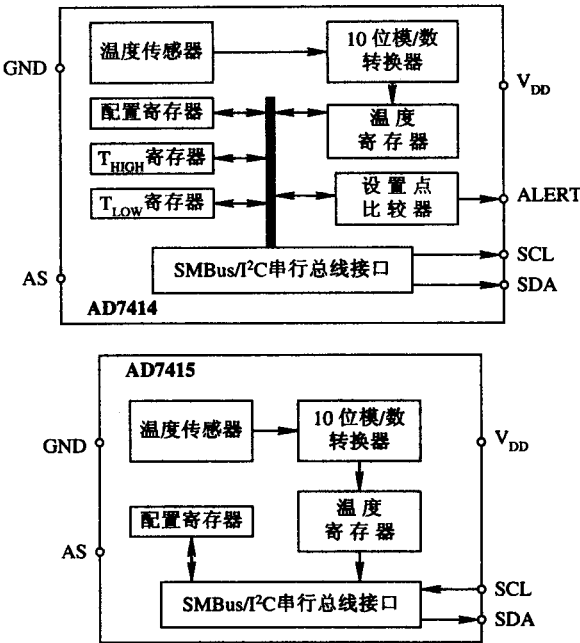
图 1.4 AD7414/AD7415 的内部原理简图
