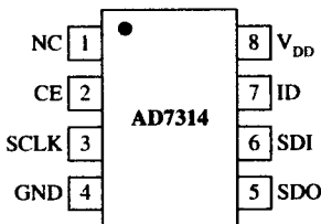
图 1.1 AD7314 的引脚图
