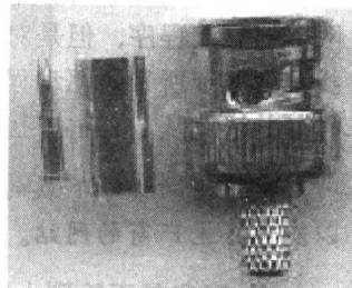
图 1-6 BNC 接头
