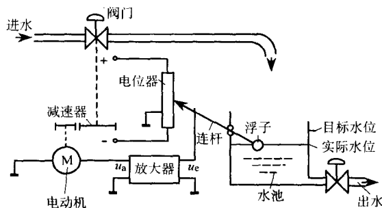
图 1-4 水位自动控制系统
