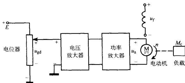
图 1-5 直流电动机转速开环控制系统
