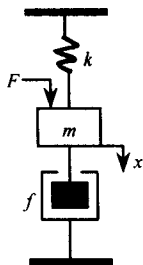
图 2-1 弹簧-质量-阻尼器系统
