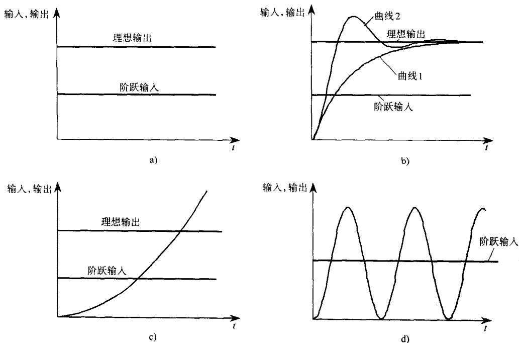
图 1-9 自动控制系统的输出响应
