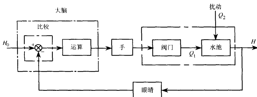
图 1-2 人工水位恒定控制系统原理框图
