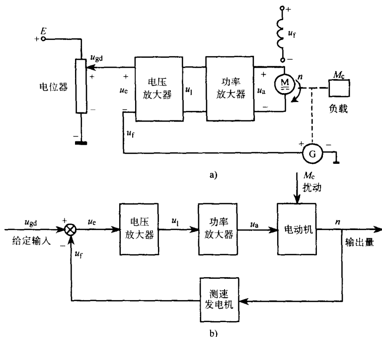
图 1-6 直流电动机转速反馈的闭环控制系统
