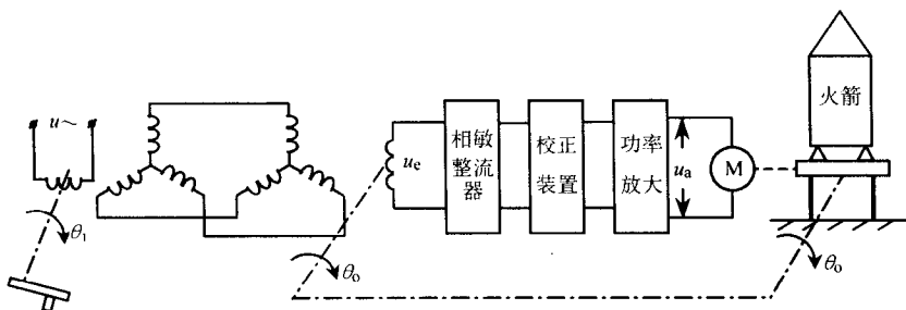
图 1-8 火箭方位角随动控制系统
