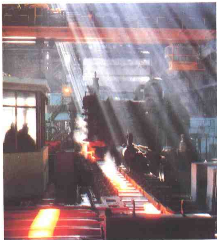
△莱钢 750 初轧生产线
