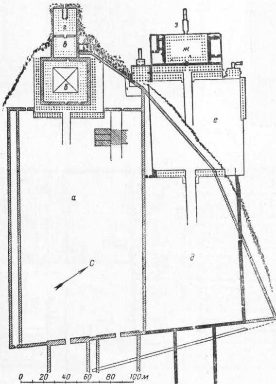
弟·埃·巴哈利建筑群 总平面
