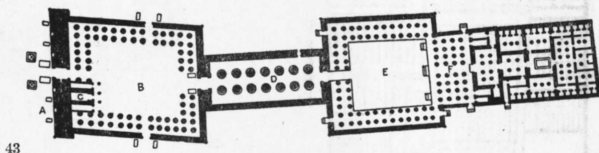
阿 蒙 神 庙 卢克索 (Luxor) 底比斯 十八王朝 約公元前 1400 年 260 × 55 米
