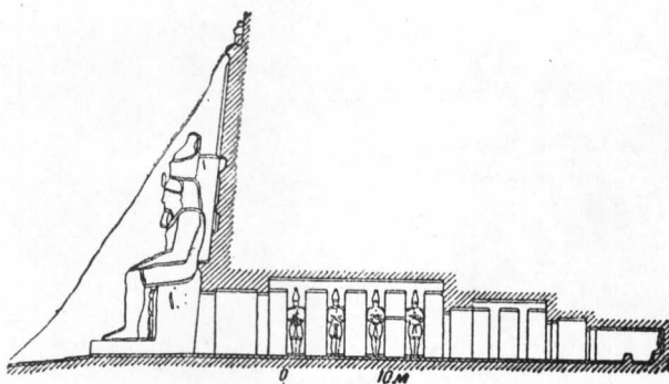
大神庙阿蒙石窟 剖面
