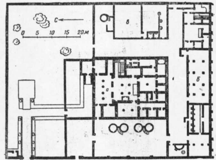
阿克塔頓城富人住宅 平 面
