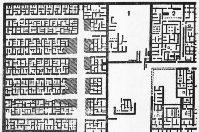
卡宏城 西北部份平面 (Kahun)
