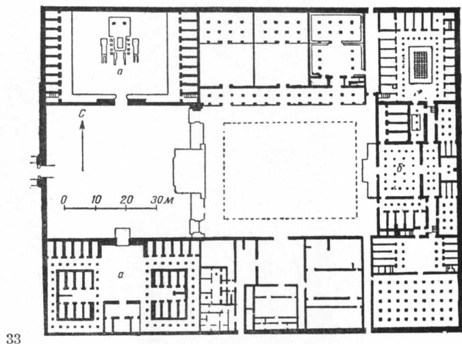
夏 宫 平 面
