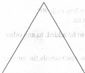
锐角三角形
