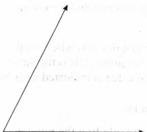
锐角
