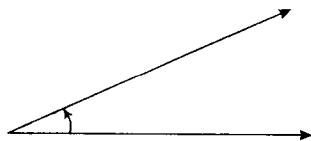
仰角
