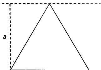
高度
