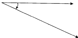
俯角
