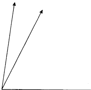
邻角
