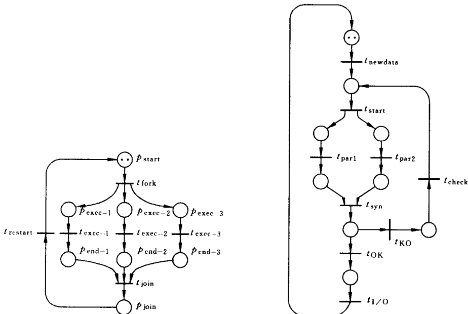
图 1.2.6 分叉和交汇操作 PN 模型
