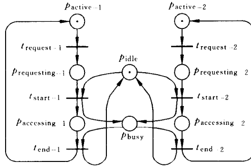
图 1.2.3 两个用户存取共享资源的 PN 模型
