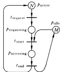
图 1.2.5 N 个用户和 M 个资源的 PN 模型
