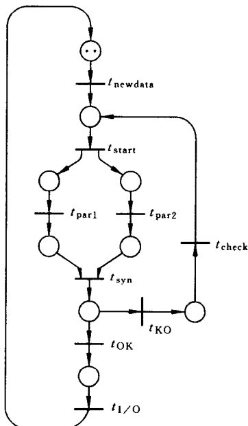
图 1.2.7 一个简单并行计算的 PN 模型
