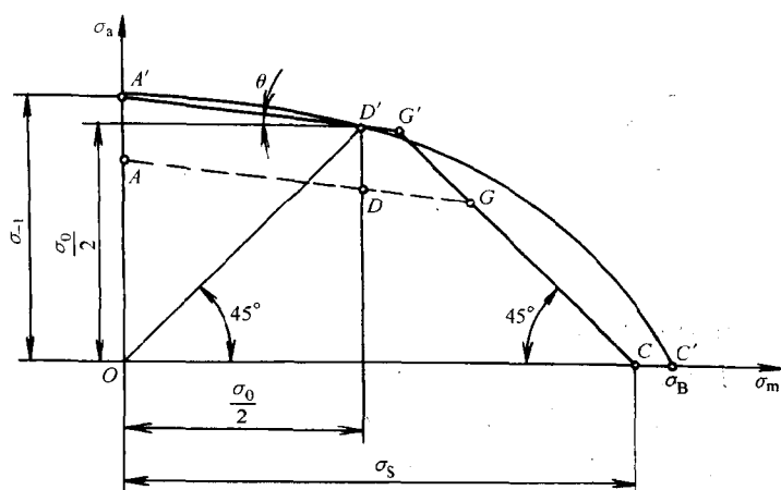
图 1-2 材料的极限应力线图
