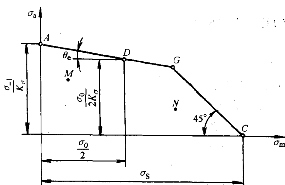
图 1-3 零件的极限应力线图
