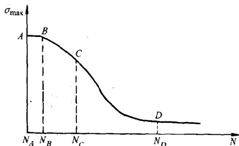
图 1-1 材料的疲劳特性曲线
