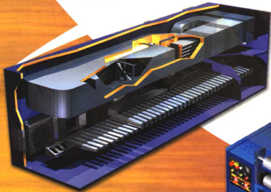
Dual Dry™ TNV 集成式的热风漂浮三区烘干机与氧化装置, 适用于高性能商业印刷。
